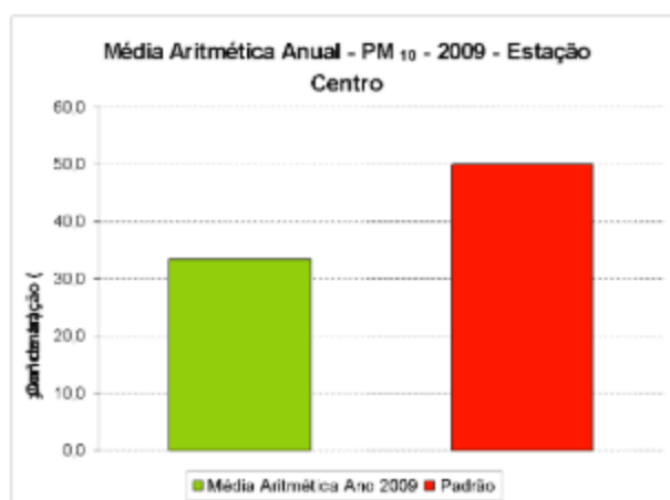
Gráfico 4 - Média aritmética dos valores de PM 10 do ano de 2009.
